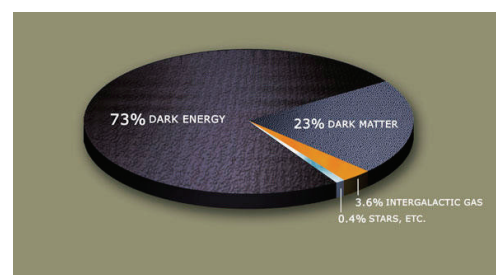
宇宙中的物質成份示意圖。觀測不到的暗物質和暗能量分別佔73%和23%（灰色部份），剩下的0.4%是發出可見光和不可見射線的星球（淺藍色），還有3.6%的星際氣體（黃色）可以通過譜線吸收觀測到。
